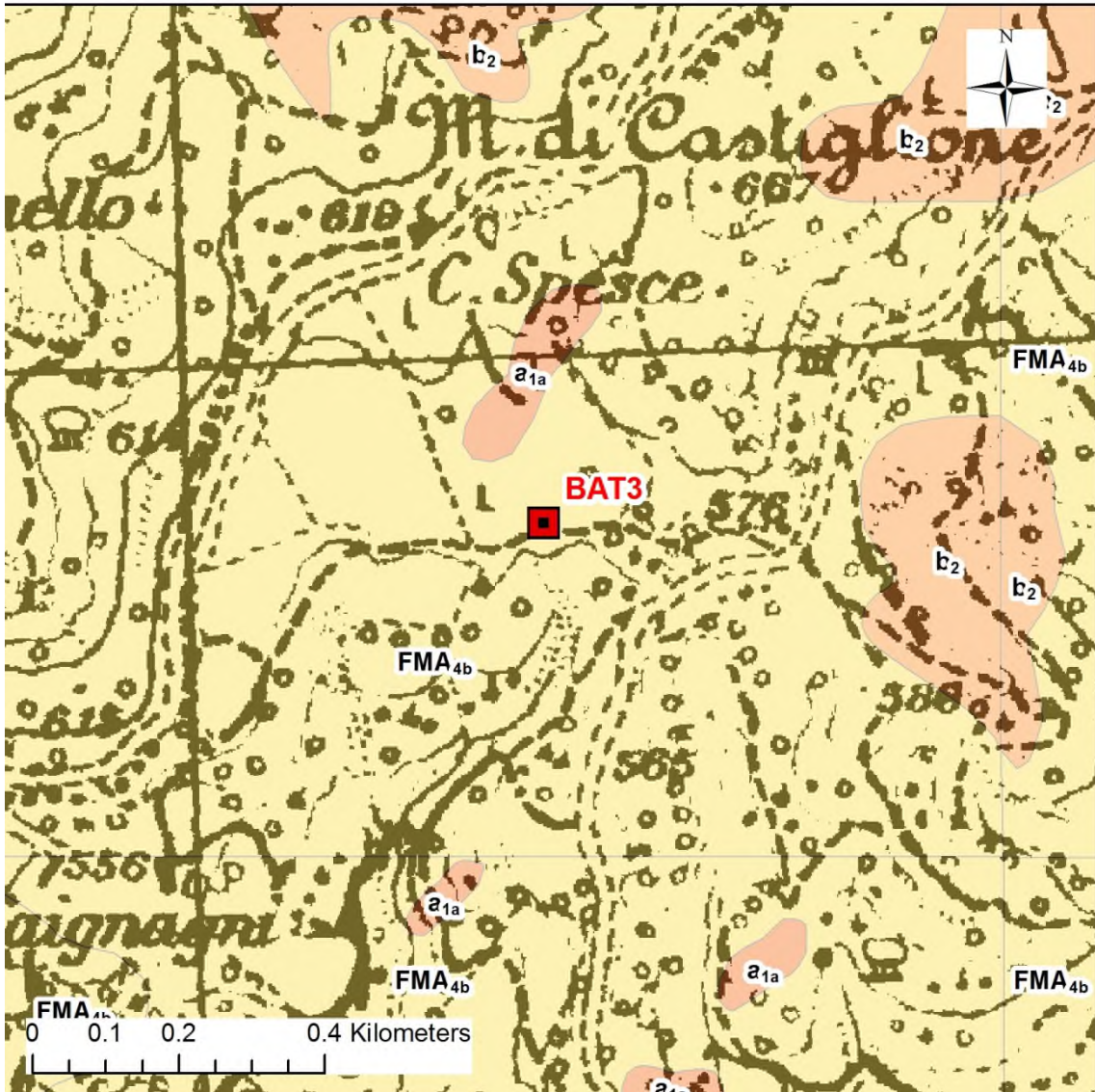
Stralcio in scala 1:10.000 della Sezione n. 290130 della Carta Geologica della Regione Umbria con l'ubicazione della Stazione Sismica.
